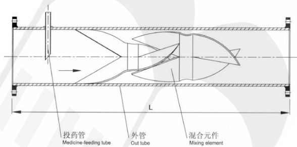
管式混合器外形图
