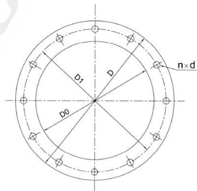
进出口法兰尺寸
